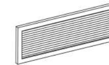
POLYCARBONATE PANEL DPP - 4530 450(L) x 18(W) x 300(H) DPP - 9030 900(L) x 18(W) x 300(H) DPP - 1230 1200(L) x 18(W) x 300(H)
