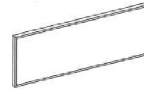
FABRIC PANEL DPP - 4530 450(L) x 18(W) x 300(H) DPP - 9030 900(L) x 18(W) x 300(H) DPP - 1230 1200(L) x 18(W) x 300(H)
